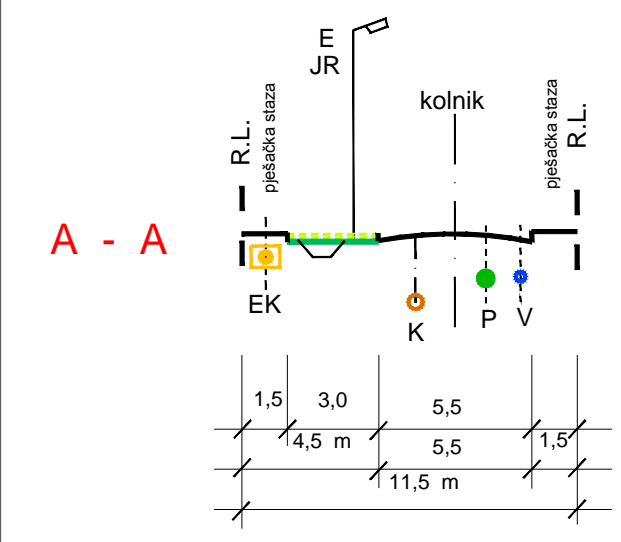
POPREČNI PRESJECI mj 1:250 (s orijentacionim elementima presjeka)
