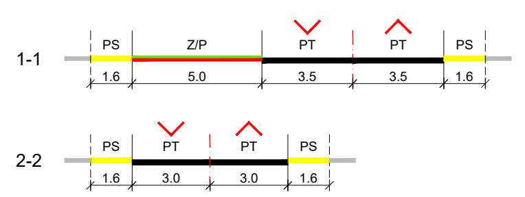
KARAKTERISTIČNI PROFILI PROMETNICA (M 1:200)
