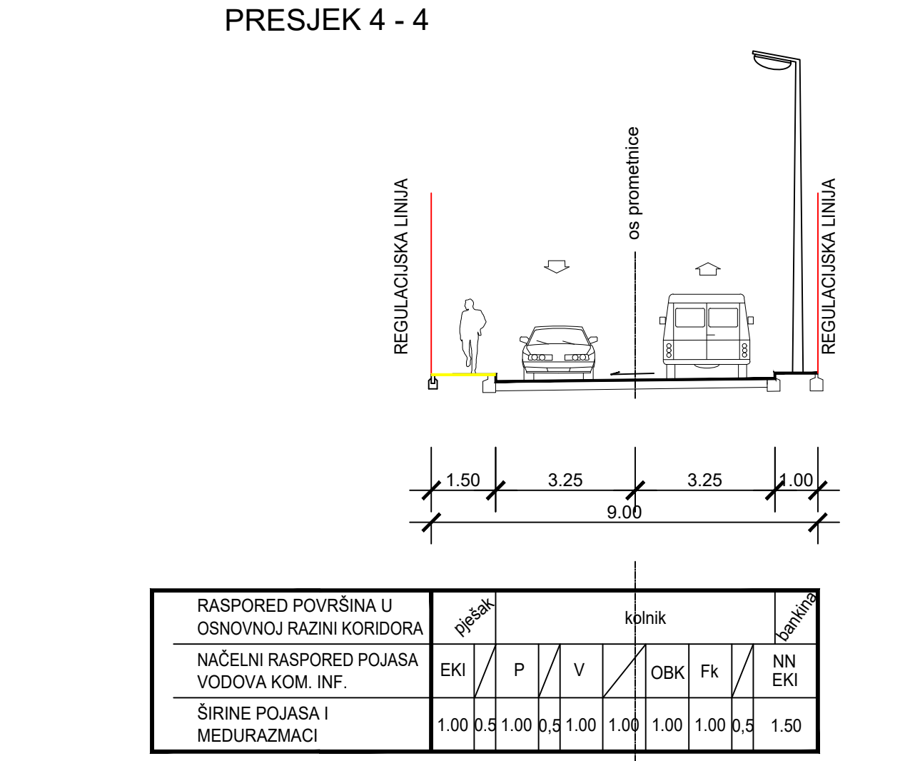
PRESJEK 4 - 4
