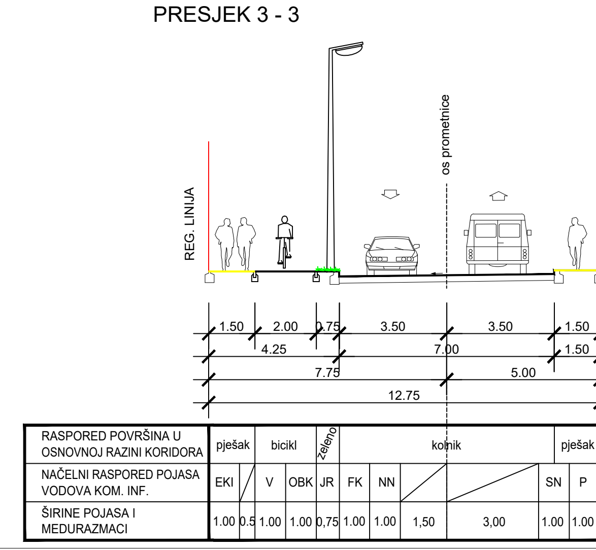
PRESJEK 3 - 3
