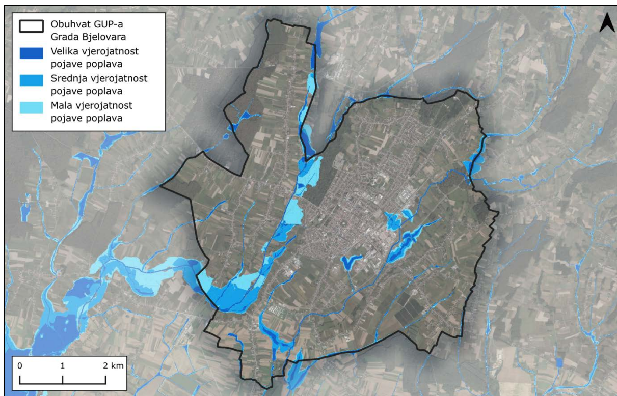
Slika 86. Opasnost od poplava prema vjerojatnosti pojavljivanja na području GUP-a u planskom ciklusu 2022.–2027. g.
