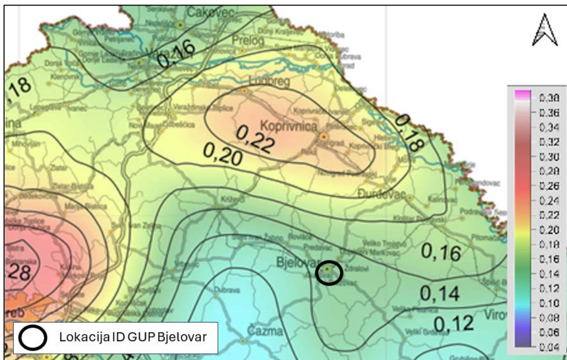
Slika 69. Kartografski prikaz potresne opasnosti za povratno razdoblje od 475 godina
