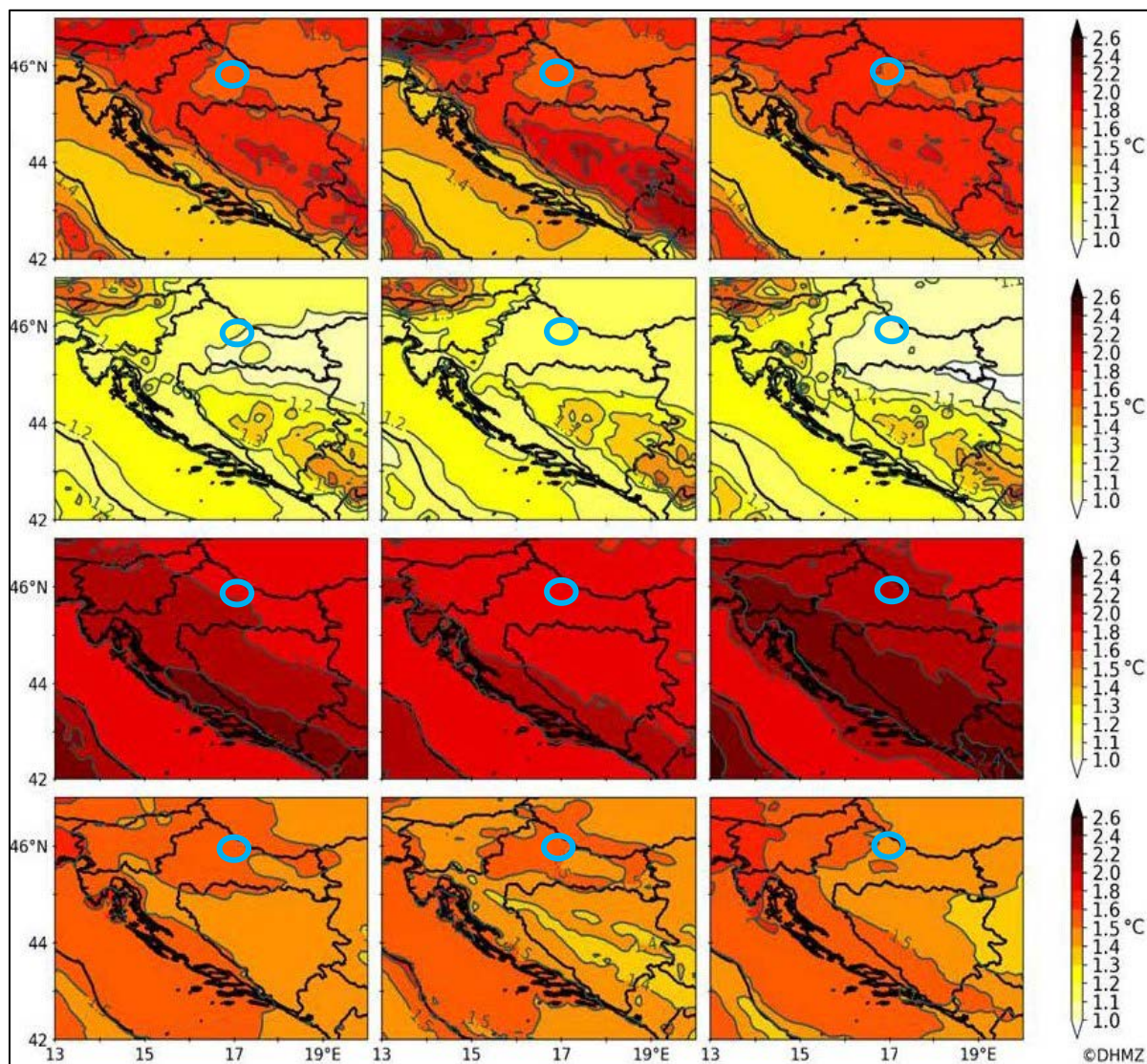
Slika 73. Sezonska promjena srednje temperature zraka na 2 m iznad tla (°C) u srednjaku ansambla modela za razdoblje 2041. - 2070. u odnosu na referentno razdoblje 1981. - 2010. godine za scenarij RCP4.5. Od lijeva na desno: srednja, minimalna, maksimalna promjena temperature zraka. Od odozgo prema dolje: zima, proljeće, ljeto, jesen
