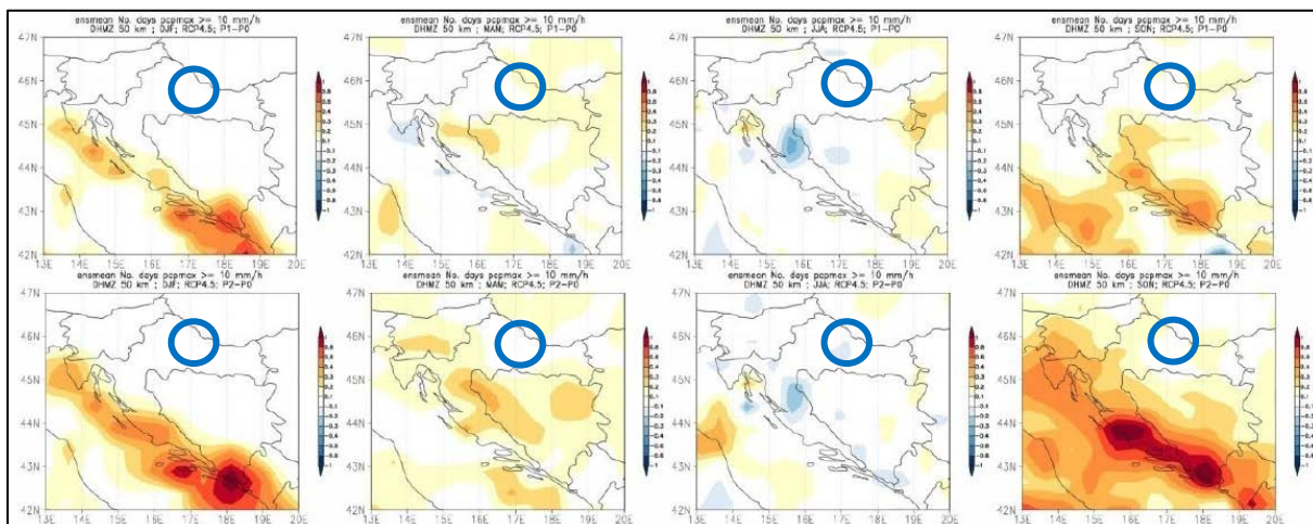
Slika 76. Broj dana s oborinom većom od 10 mm/h u srednjaku ansambla iz četiri integracije RegCM modelom. Od lijeva na desno: zima, proljeće, ljetu i jesen. Gore: promjena u razdoblju 2011.-2040.; dolje: promjena u razdoblju 2041.-2070.
