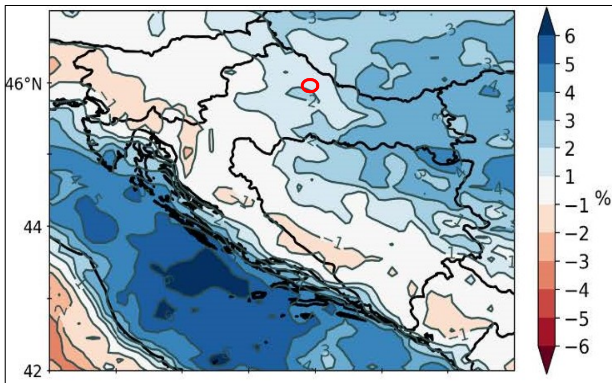
Slika 74. Relativna promjena ukupne srednje količine oborine u srednjaku ansambla korištenih modela za razdoblje 2041. - 2070. u odnosu na referentno razdoblje 1981. - 2010. godine za scenarij RCP4.5.
