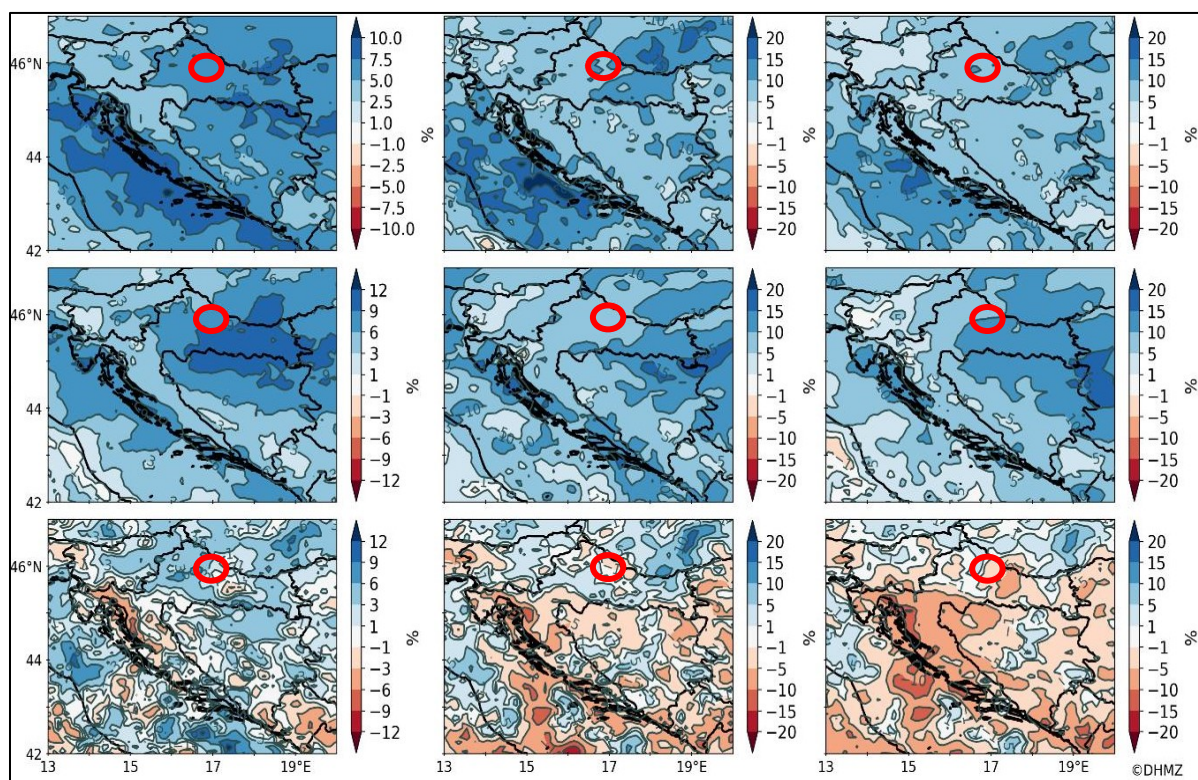
Slika 81. Relativna promjena standardnog dnevnog intenziteta oborine, najveće 1-dnevne količine oborine i najveće 5-dnevne količine oborine u srednjaku ansambla korištenih modela za razdoblje 2041. - 2070. u odnosu na referentno razdoblje 1981. - 2010. godine za scenarij RCP4.5. Od odozgo prema dolje: godišnja promjena, promjena zimi, promjena ljeti. Lijevi stupac: standardni dnevni intenzitet oborine, srednji stupac: 1-dnevna količina oborine, desni stupac: 5-dnevna količina oborine
