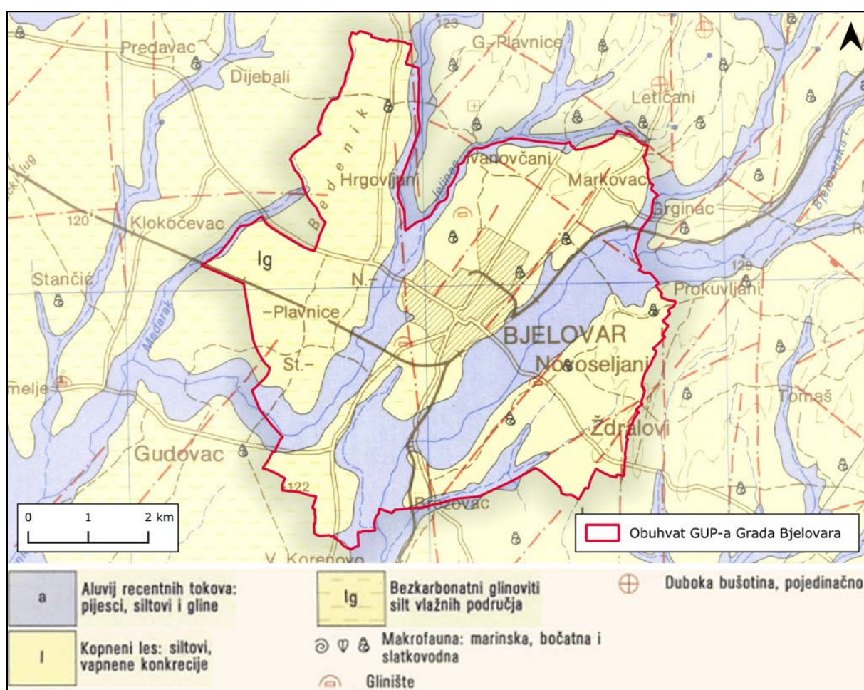
Slika 67. Isječak Osnovne geološke karte s obuhvatom GUP-a Grada Bjelovara
